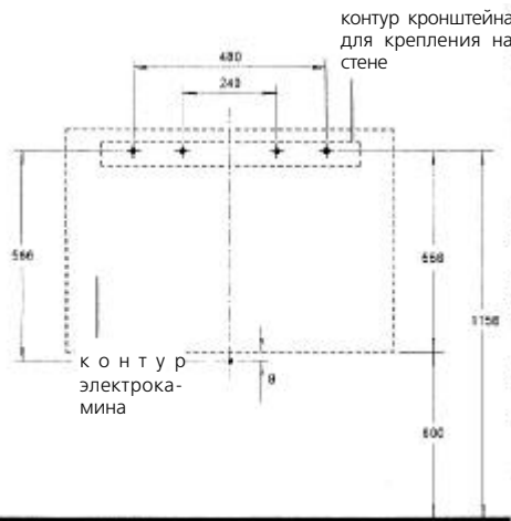
Иллюстрация 2: Рекомендуемые крепежные размеры
